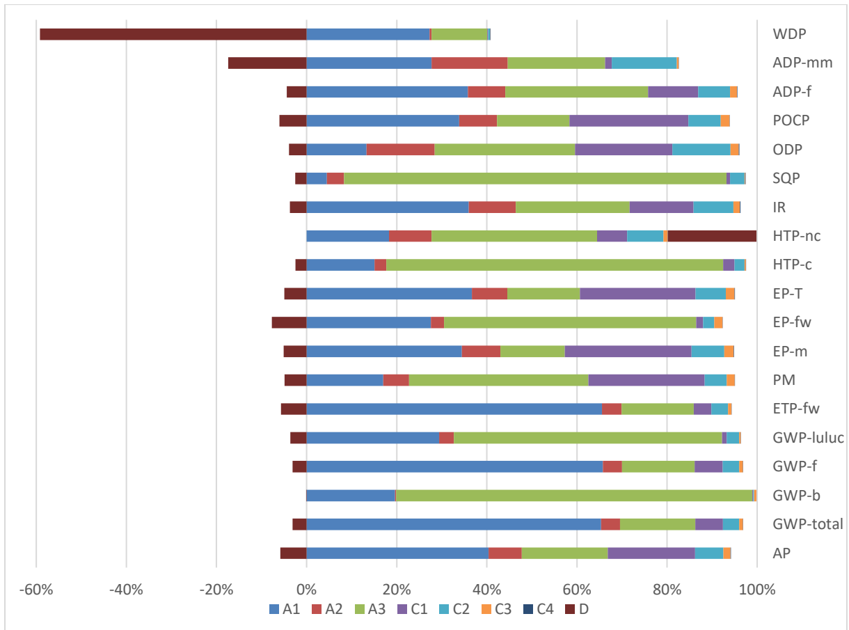
Abbildung 2: Anteile der Produktlebensphasen an den Umweltwirkungen für C50/60 selbstverdichtend
