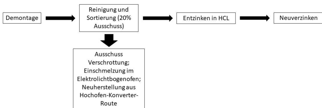
Abbildung 1: Prozessflussbild „ReUse“ Verfahren
