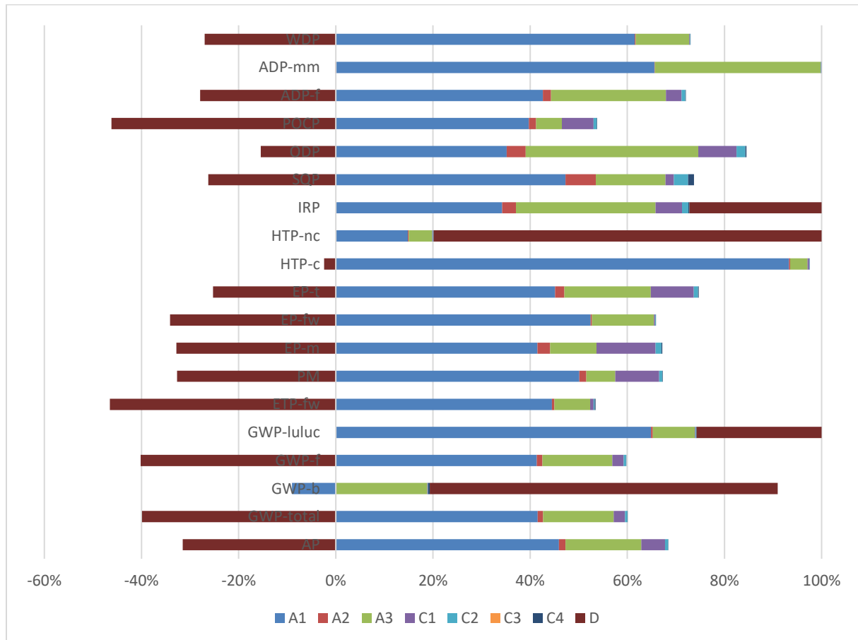
Abbildung 2: Anteile der Produktlebensphasen an den Umweltauswirkungen für 1 Tonne ReUse-Stahl
